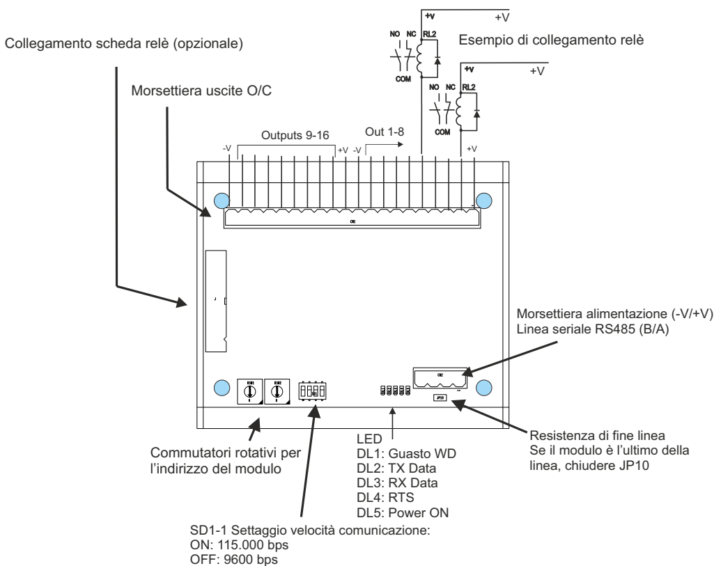
Figura 1) Topografico STG/IN8S
