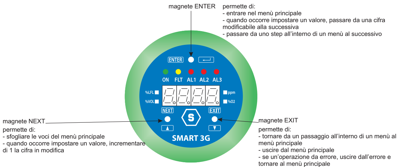
Figura 4) Utilizzo tasti ENTER, NEXT e EXIT
