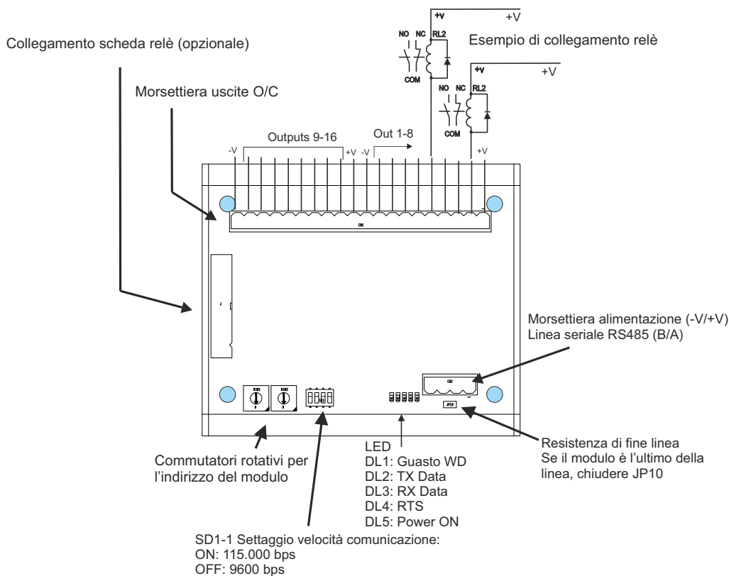
Figura 1) Topografico STG/IN8S
