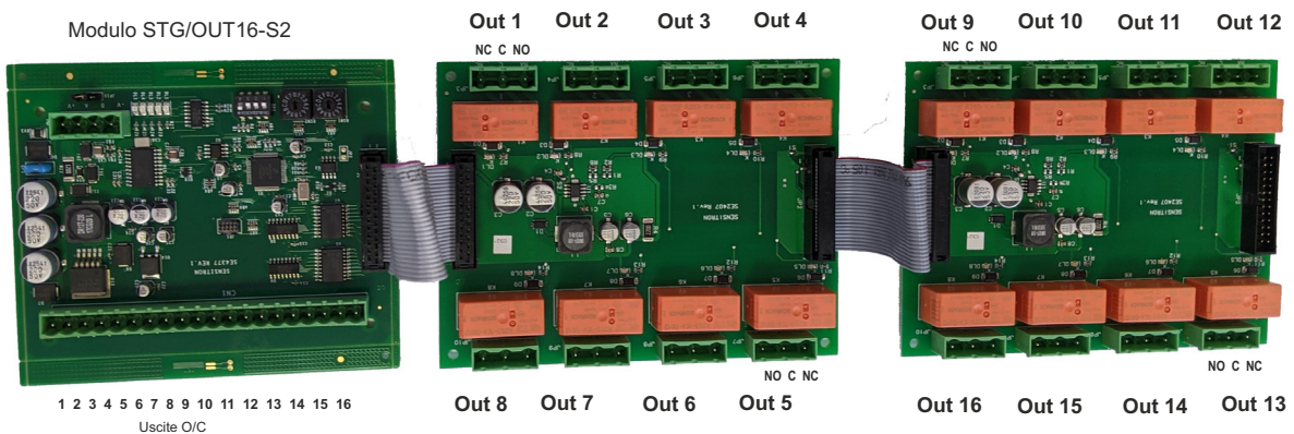
Figura 3) Collegamento scheda relè
