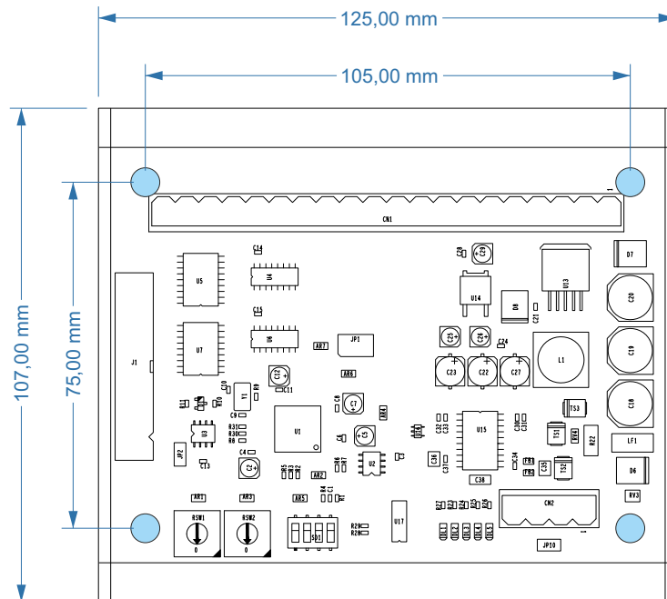
Figura 4) Dimensione modulo
