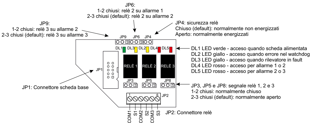
Figura 4) Scheda 3 relè
