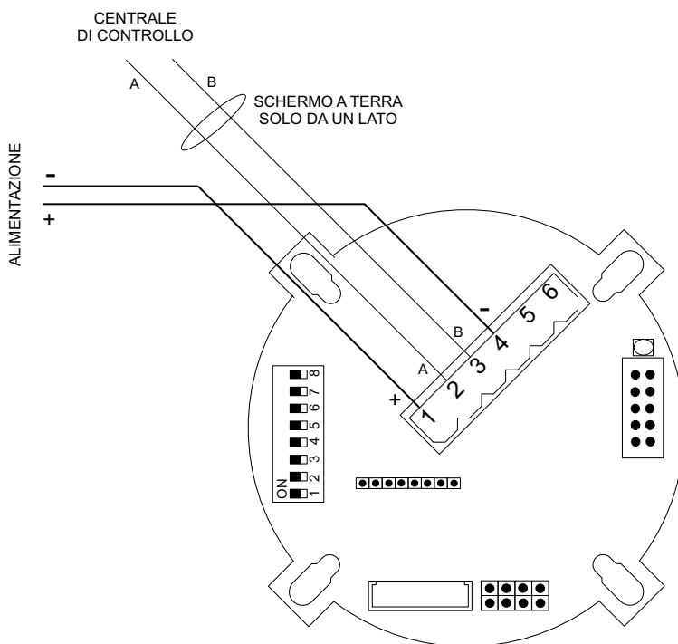
Figura 3) Collegamento rivelatore su bus seriale RS485
