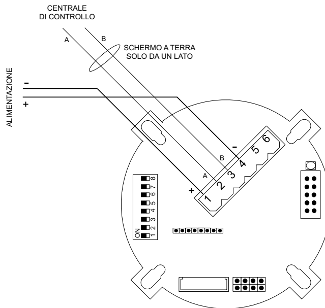
Figura 3) Collegamento rilevatore su bus seriale RS485
