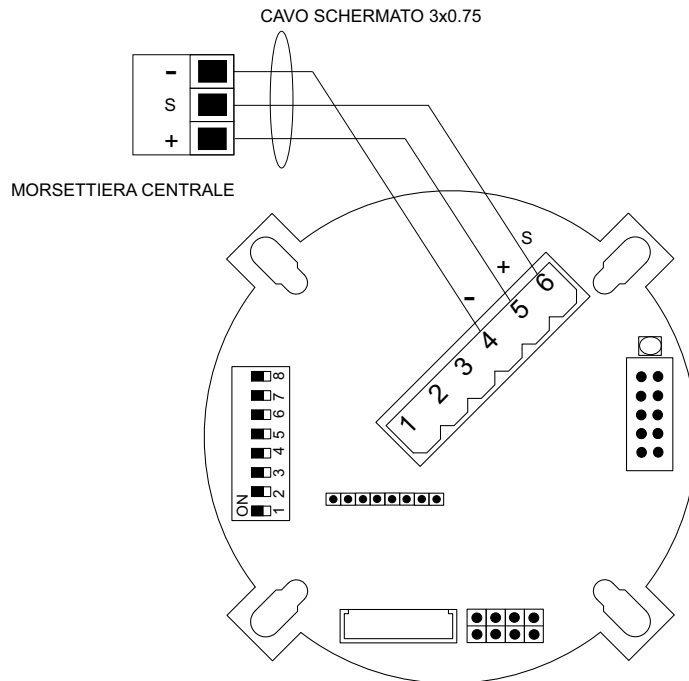
Figura 1) Schema di collegamento per l'uscita 4-20 mA con cavo schermato
