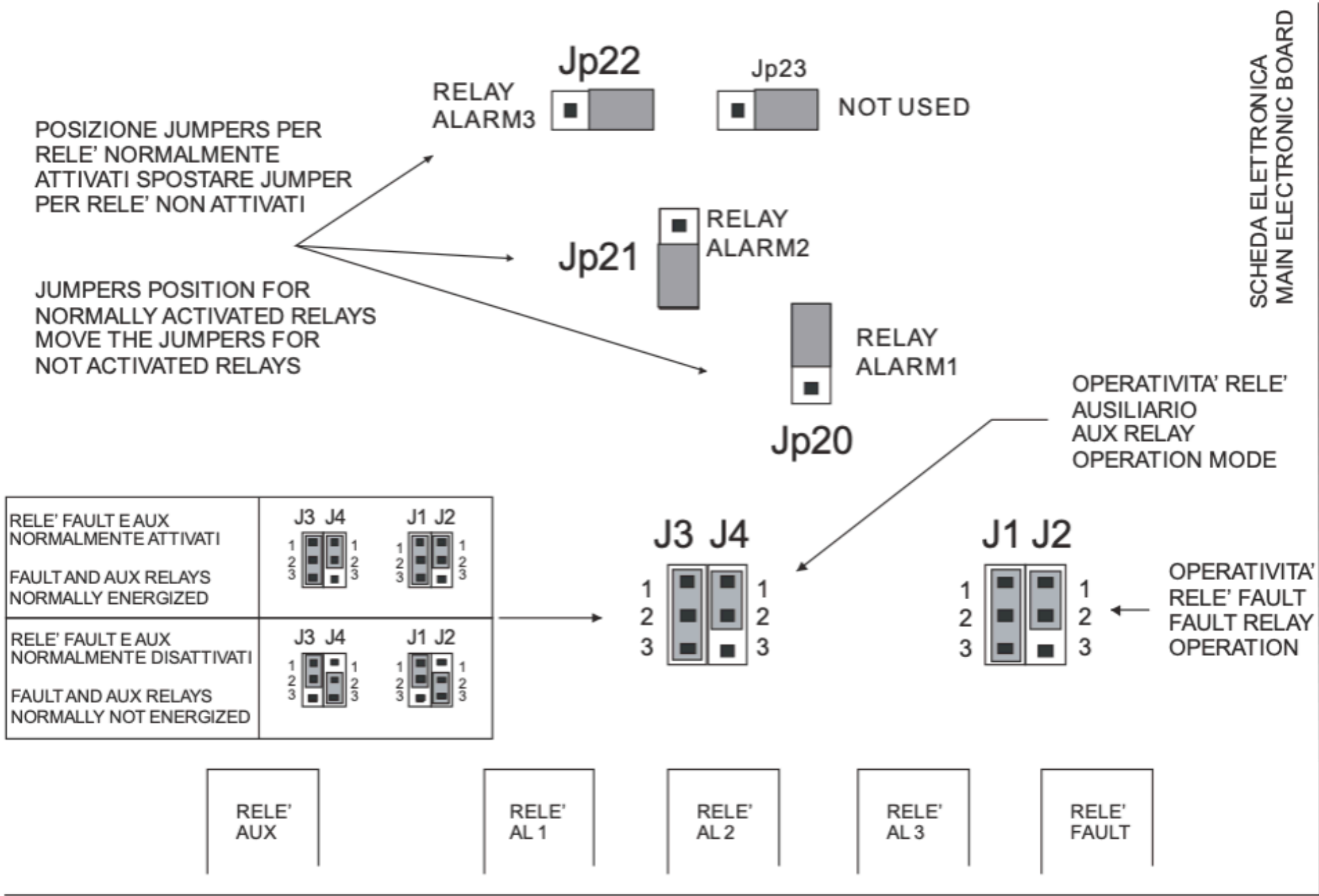
MODALITÀ OPERATIVE RELÈ
