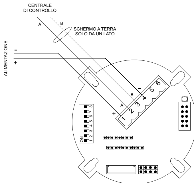
Figura 3) Collegamento rilevatore su bus seriale RS485
