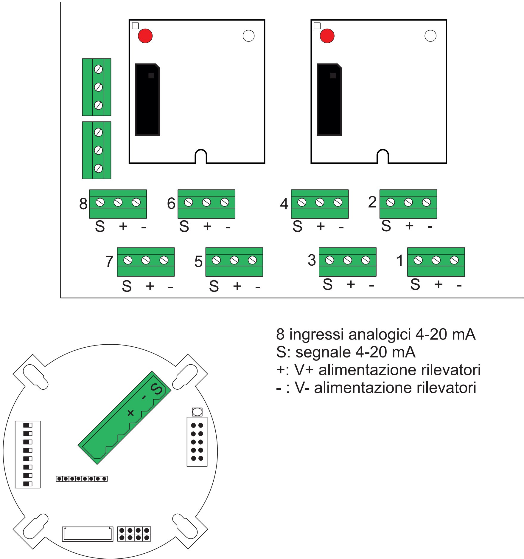
Figura 10 Collegamento degli 8 rilevatori in centrale
