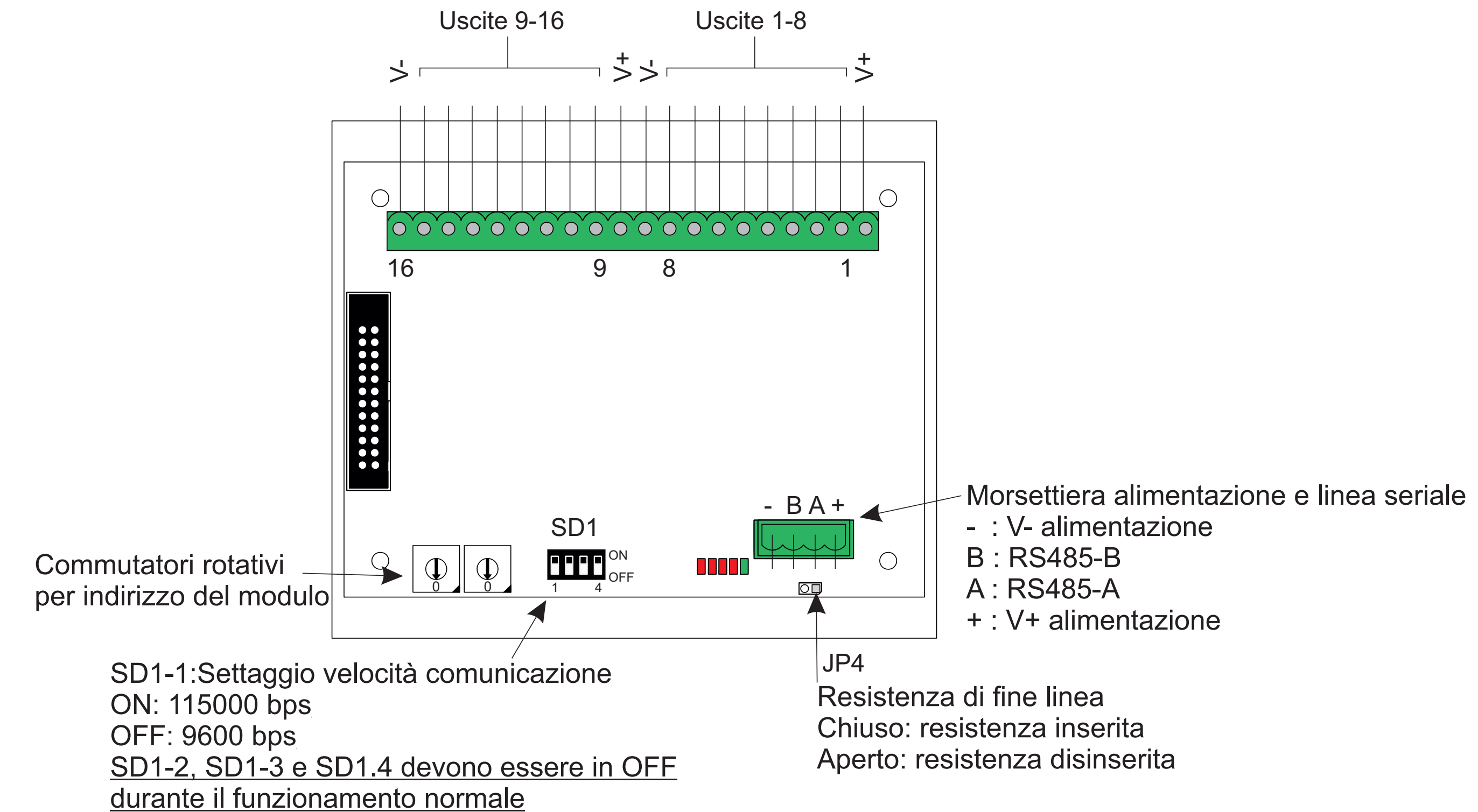
Figura 14 Modulo STG/OUT16S
