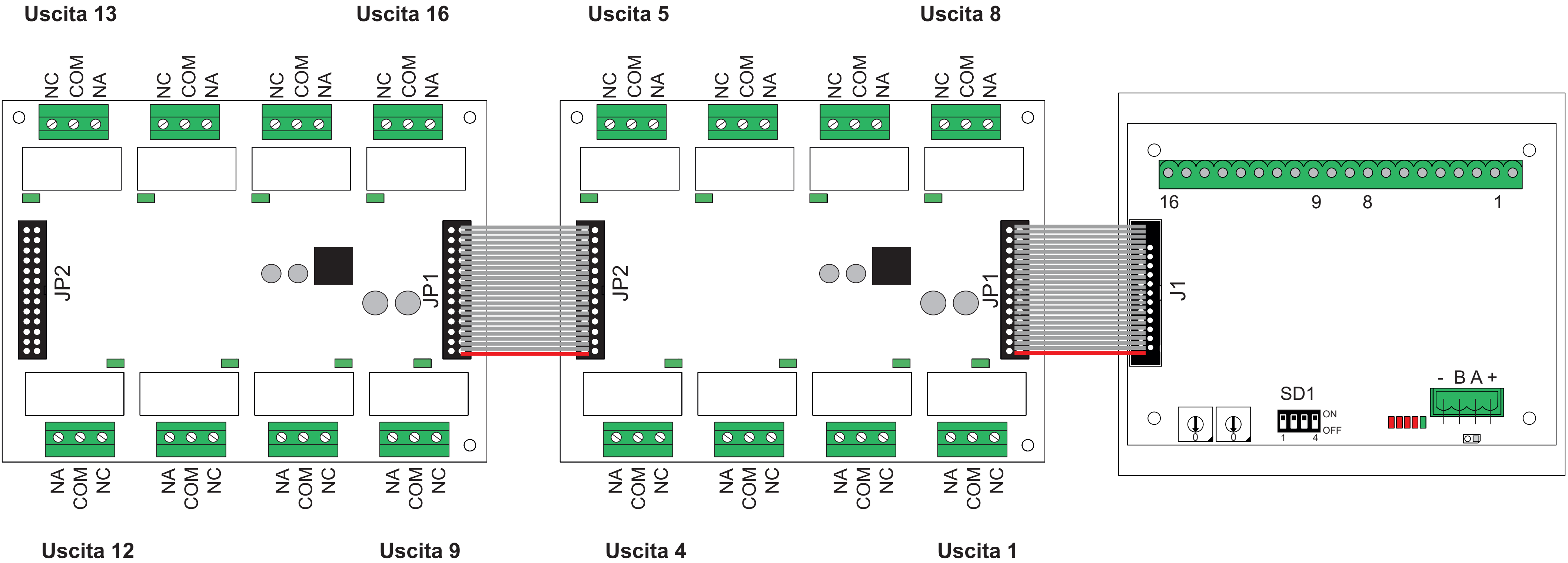
Figura 15 Scheda relè e collegamento a modulo uscita
