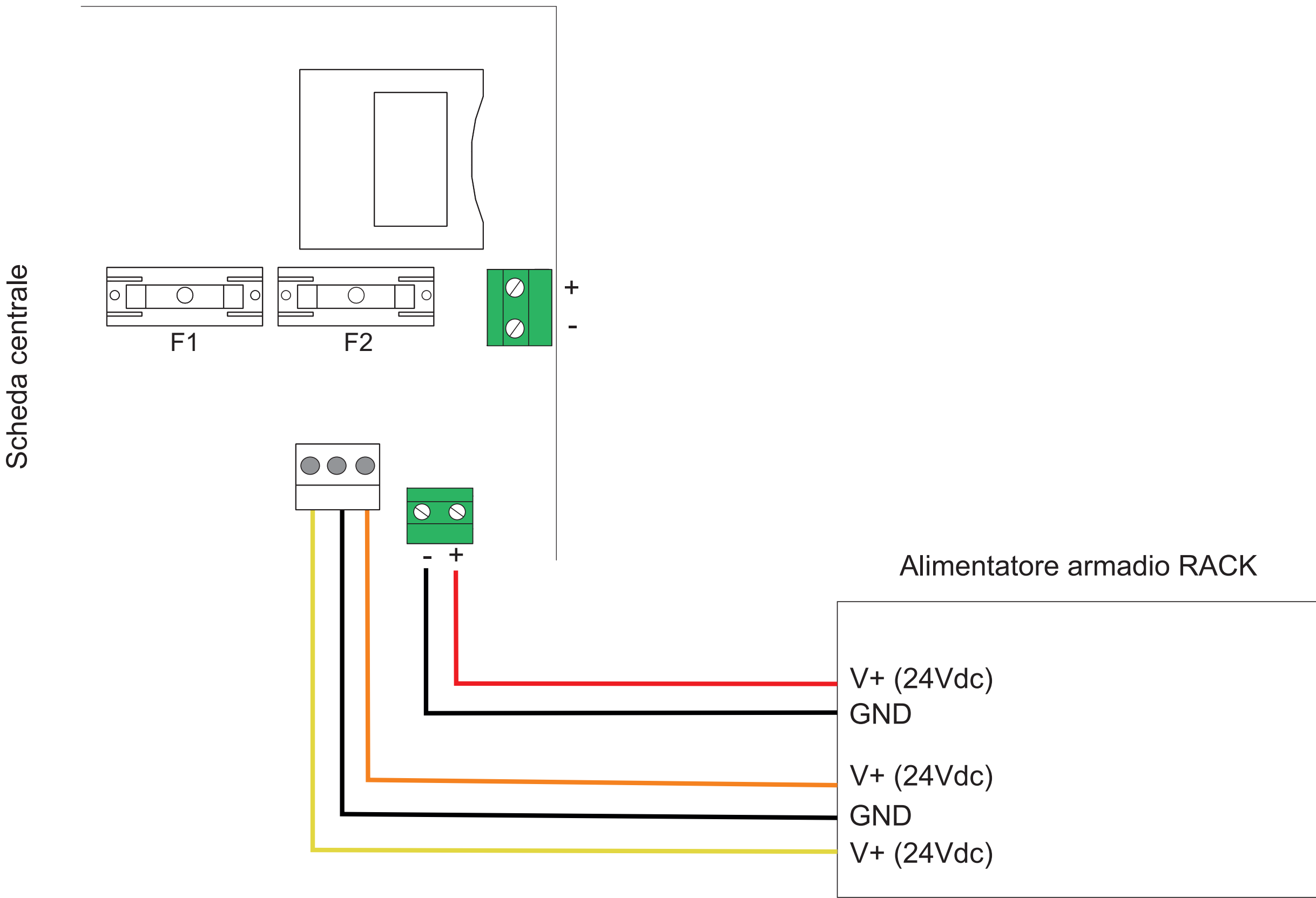
Figura 8 Collegamento alimentazione - versione rack
