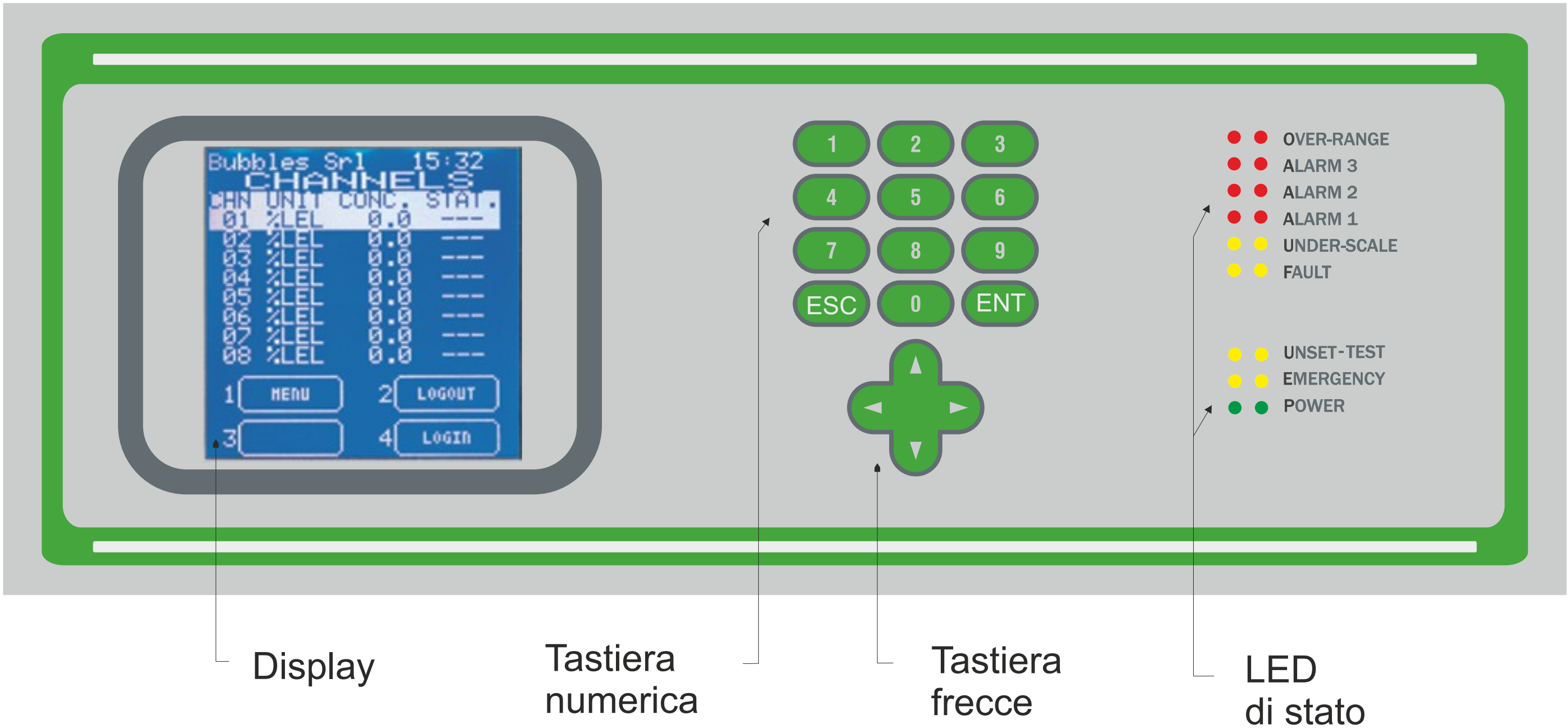
Figura 21 Pannello frontale centrale
