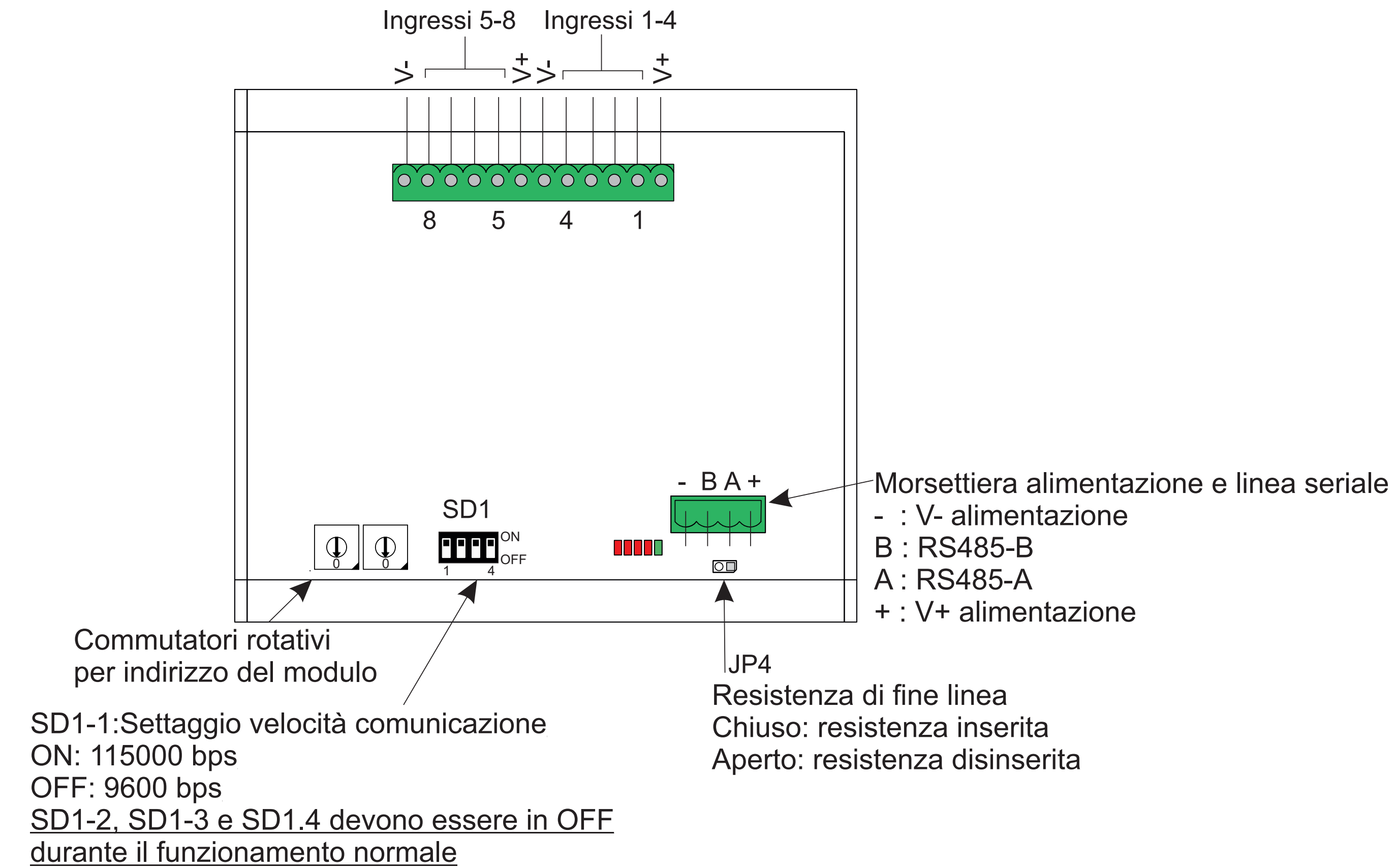
Figura 13 Modulo STG/IN8S
