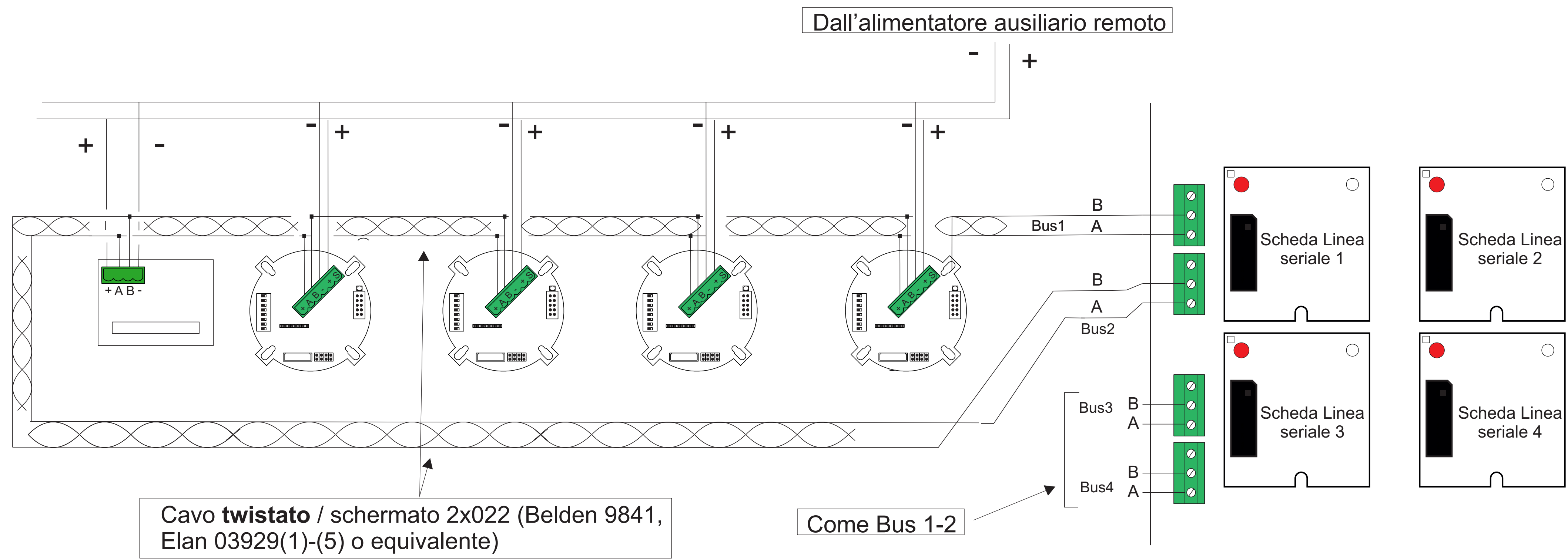
Figura 12 Collegamento dispositivi su loop RS485
