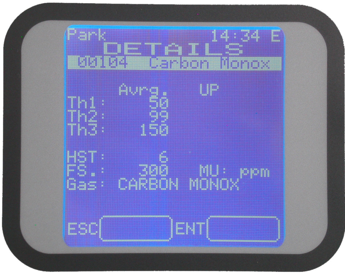
Figura 46 Dettagli configurazione rilevatore gas
