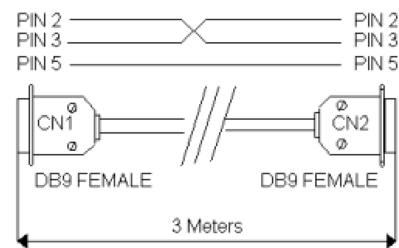
Figura 17 Cavo collegamento PC
