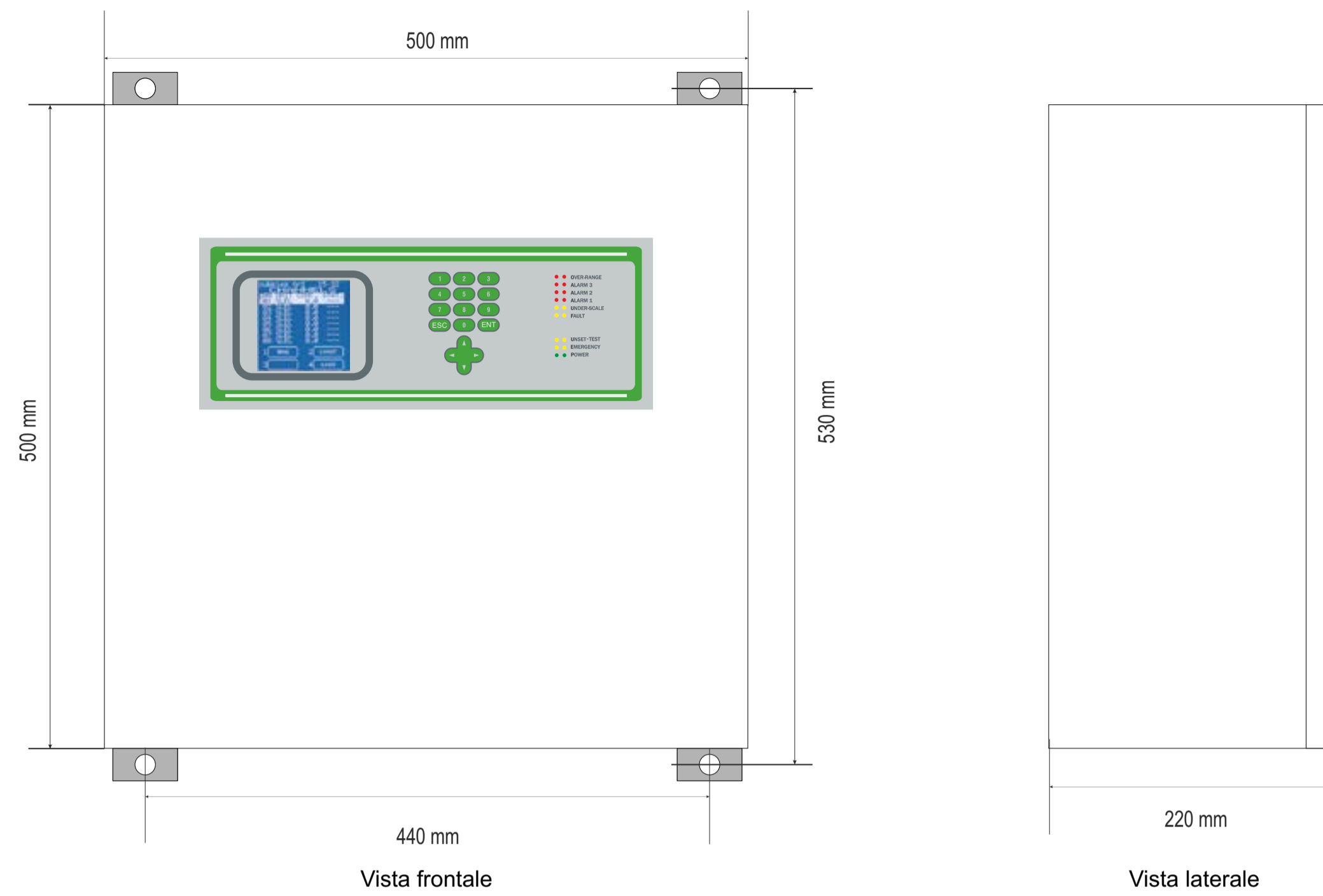
Figura 4 Dimensioni del box centrale (mm)
