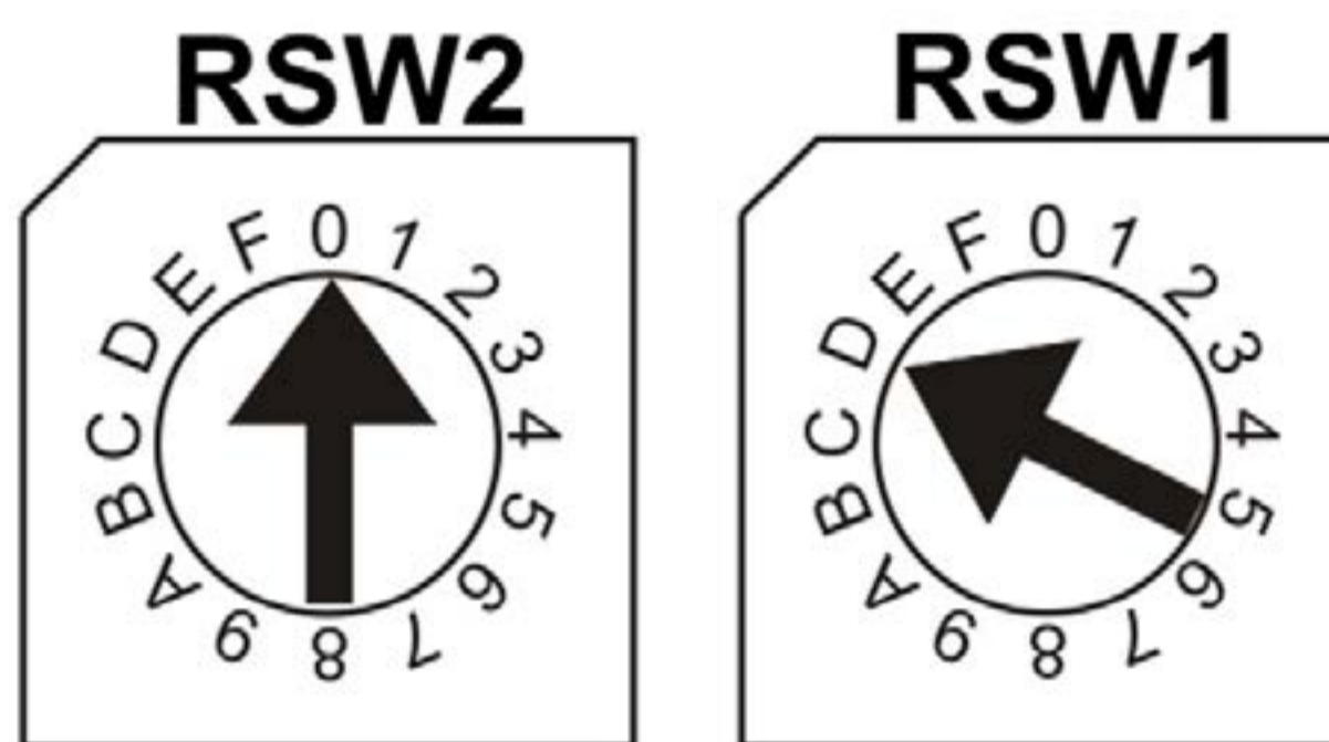
Figura 13 Esempio: Se i due commutatori sono posizionati come sopra, RSW2 su 0 ed RSW1 su D, l'indirizzo corrispondente in decimale è 13 (vedi tabella sottostante)
