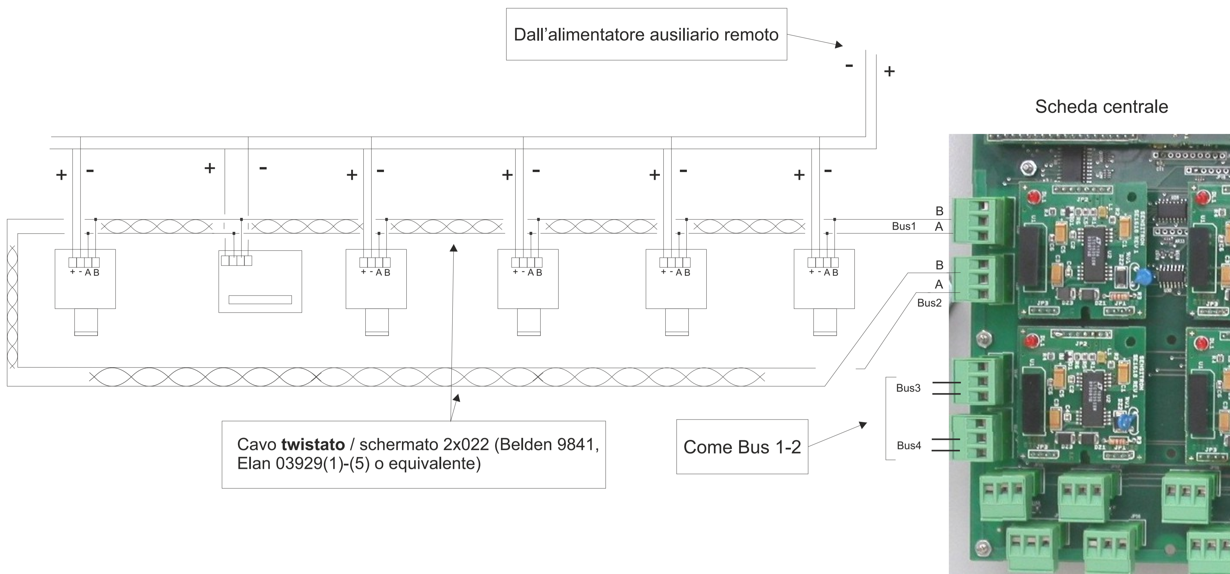
Figura 9 Collegamento dispositivi su loop RS485
