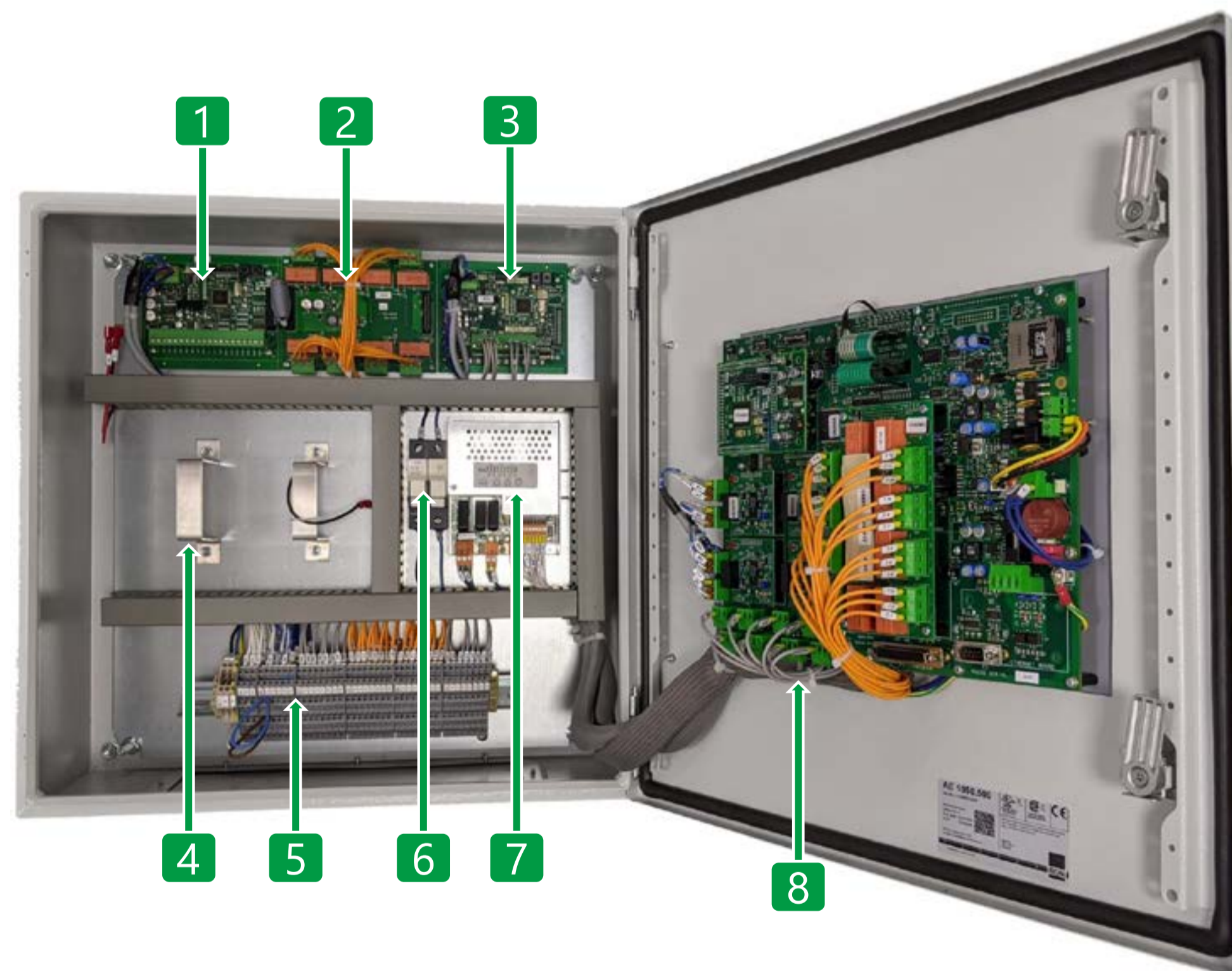
Figura 5 Vista d'assieme centrale ed identificazione delle parti
