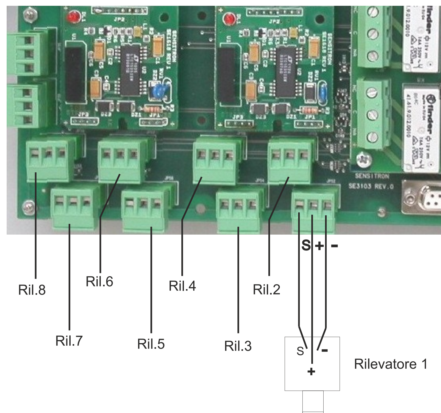
Figura 7 Collegamento degli 8 rilevatori in centrale
