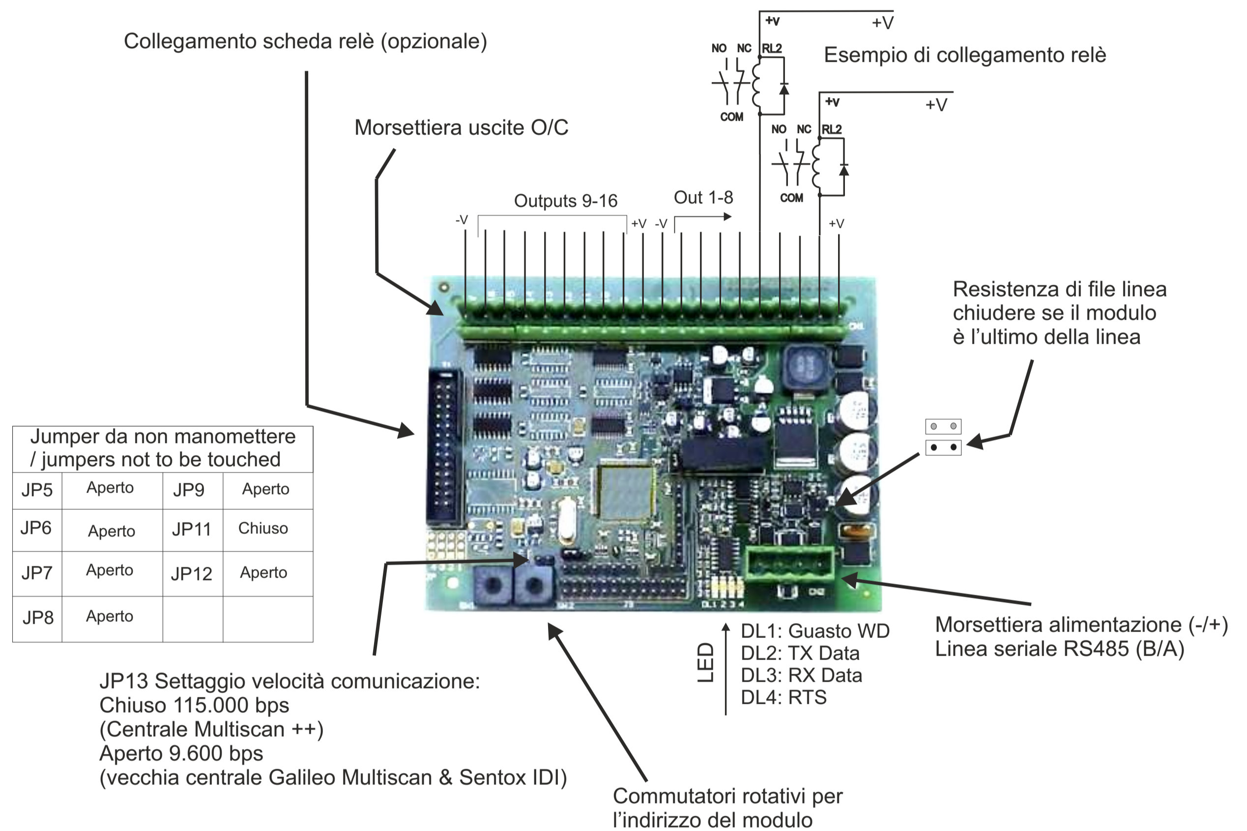
Figura 11 Modulo STG/OUT16-S2MED
