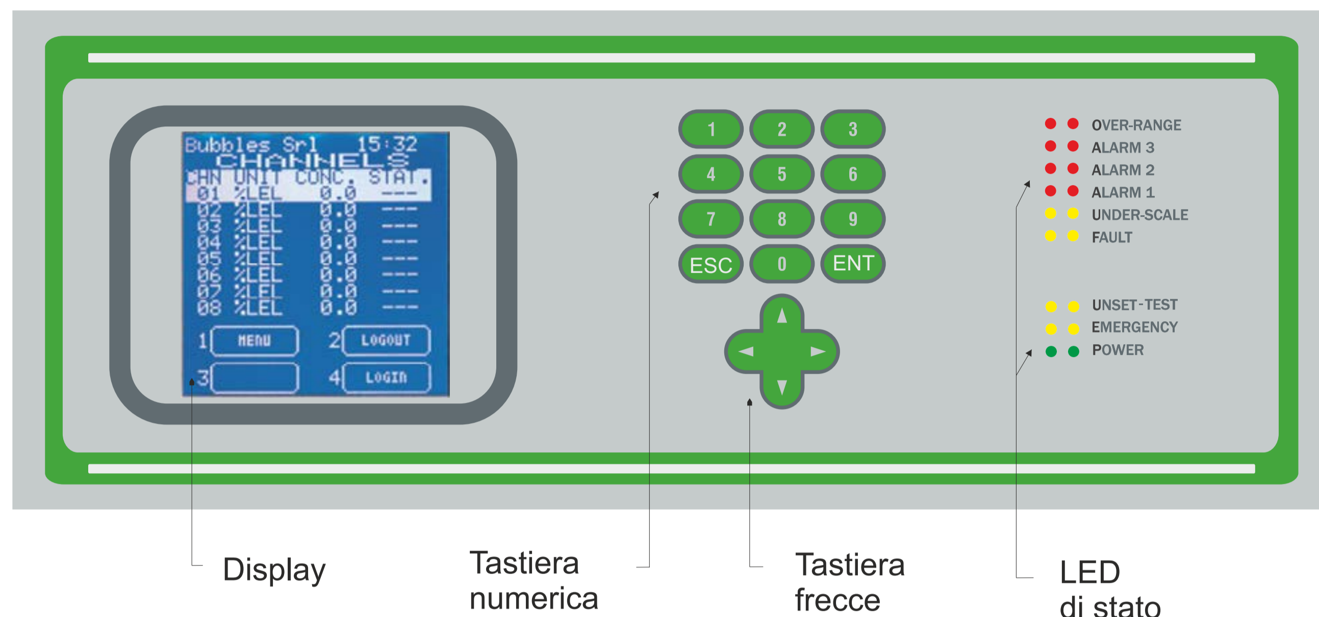
Figura 16 Pannello frontale centrale
