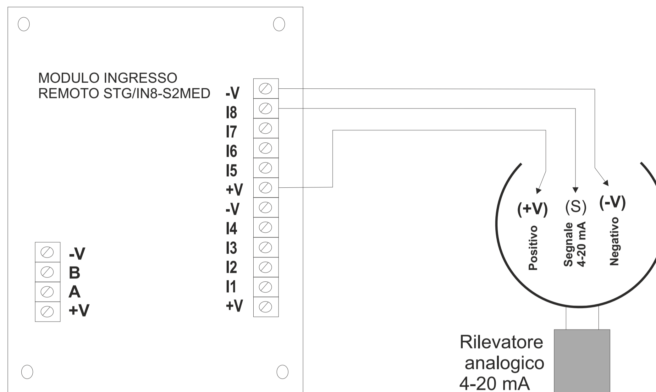
Figura 8 Collegamento degli 8 rilevatori al modulo STG/IN8-S2MED
