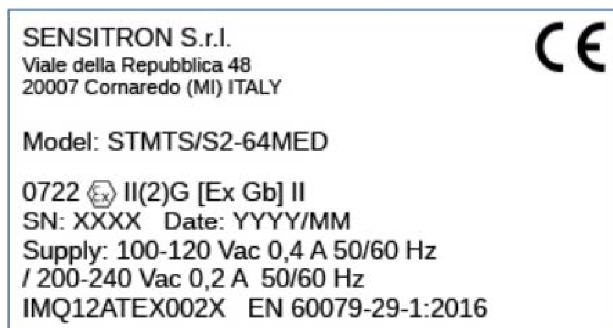
Figura 2 Esempio marcatura ATEX, centrale versione rack
