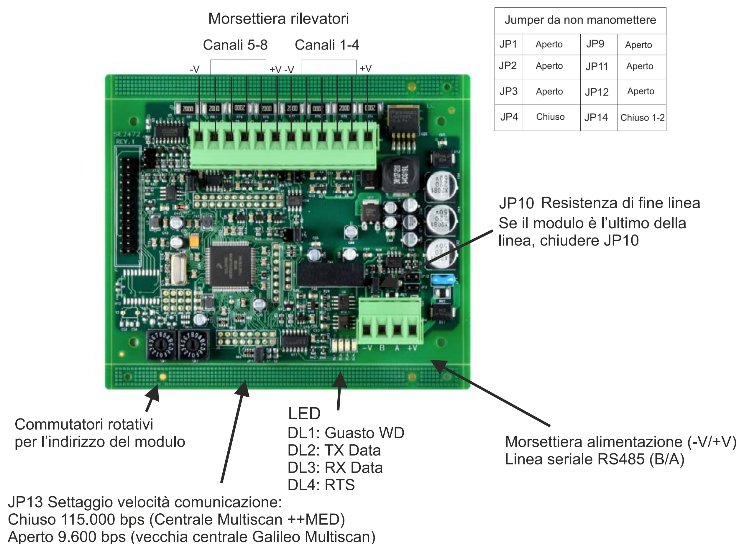
Figura 10 Modulo STG/IN8-S2MED
