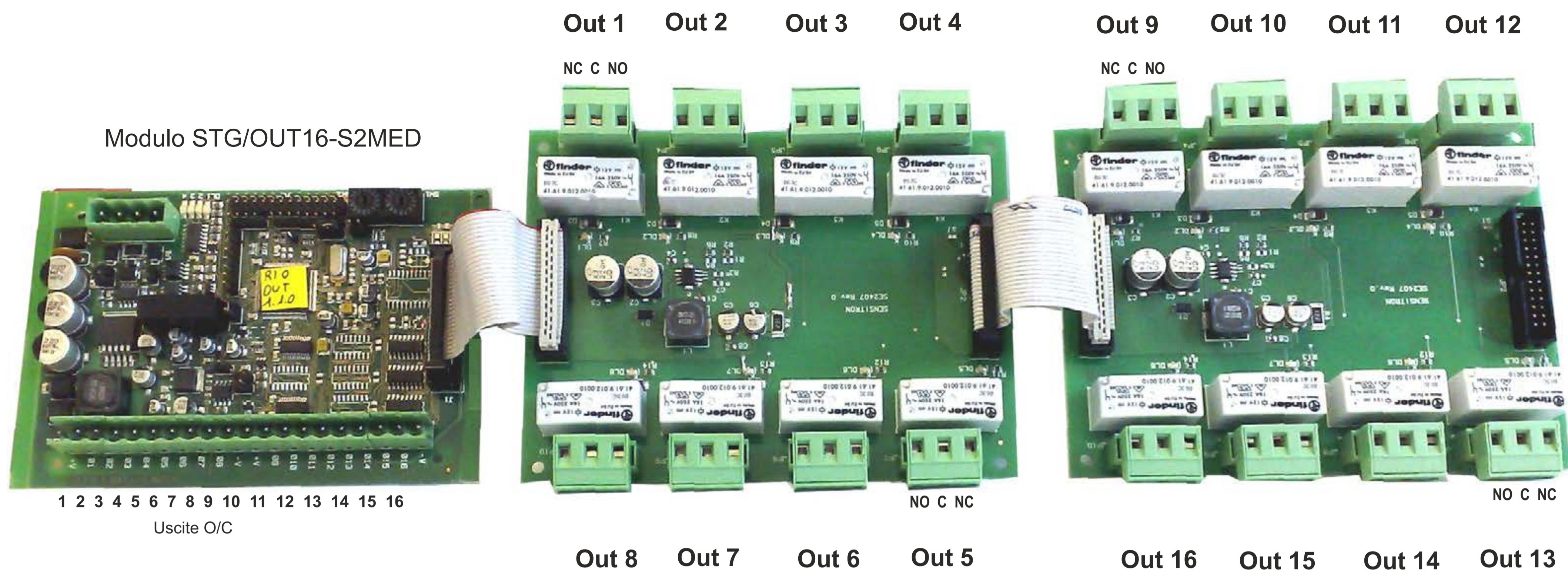
Figura 12 Scheda relè e collegamento a modulo uscita
