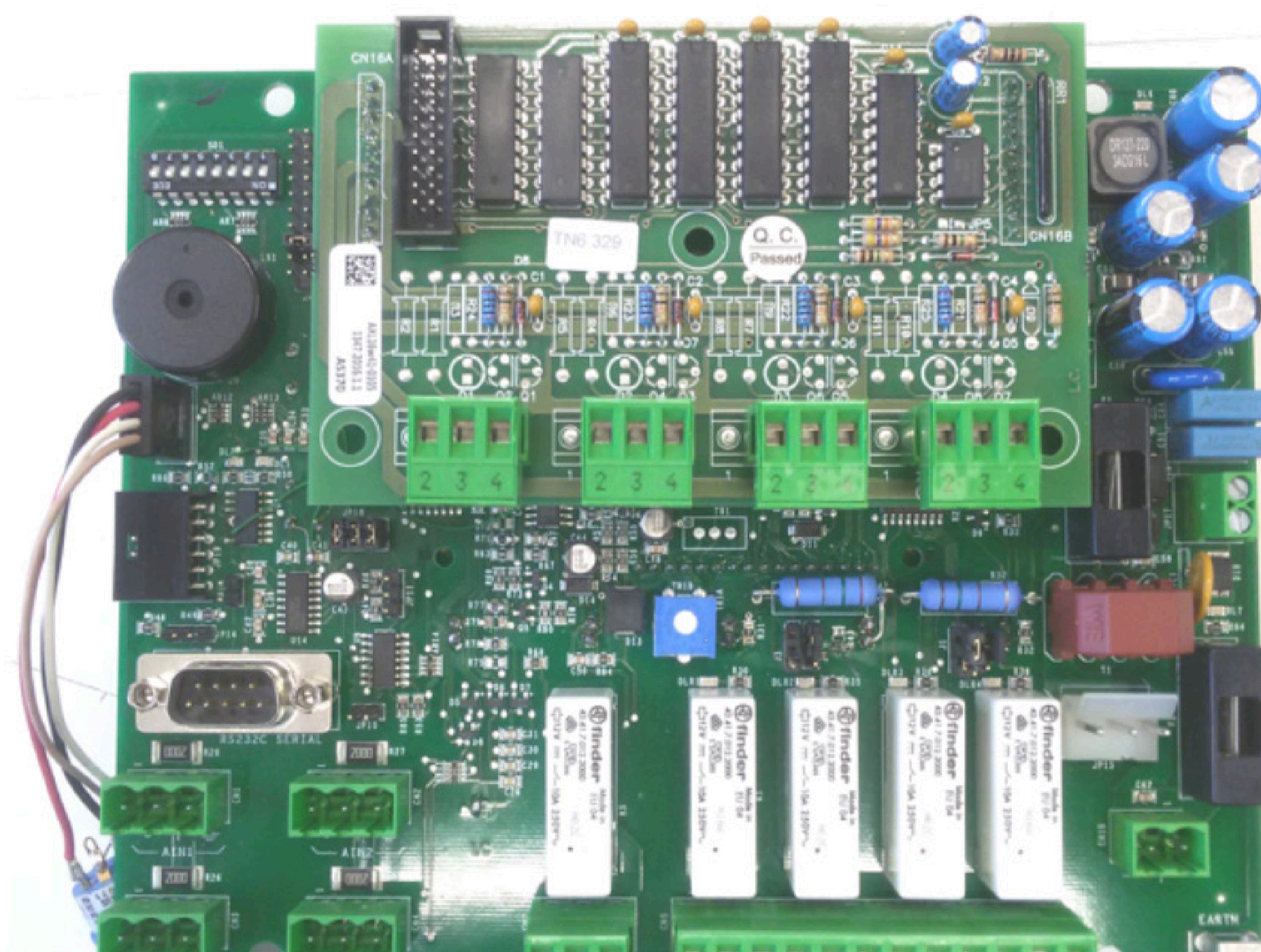
SCHEDA ESPANSIONE STPL4/ESP STPL4/ESP EXPANSION BOARD
