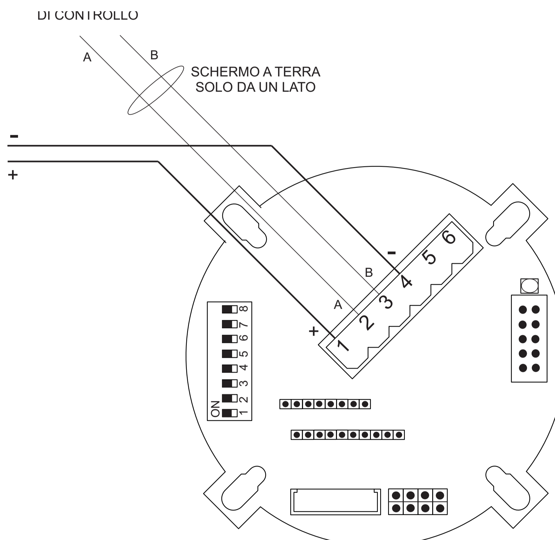
Figura 3: Collegamento rivelatore su bus seriale RS485
