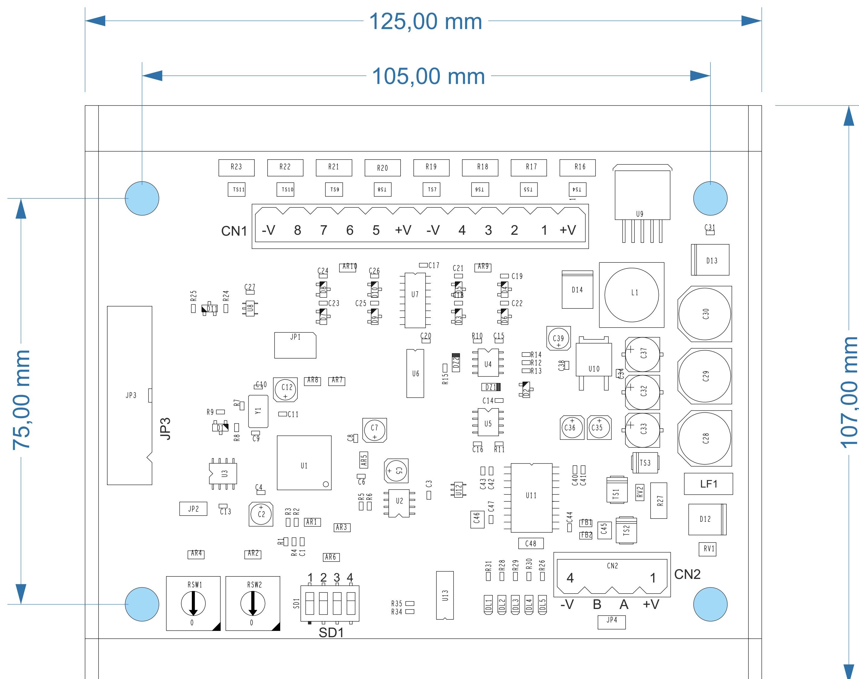
Fig.4 Dimensione modulo, misure in millimetri
